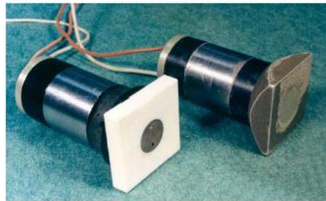
Terfenol-D actuators
